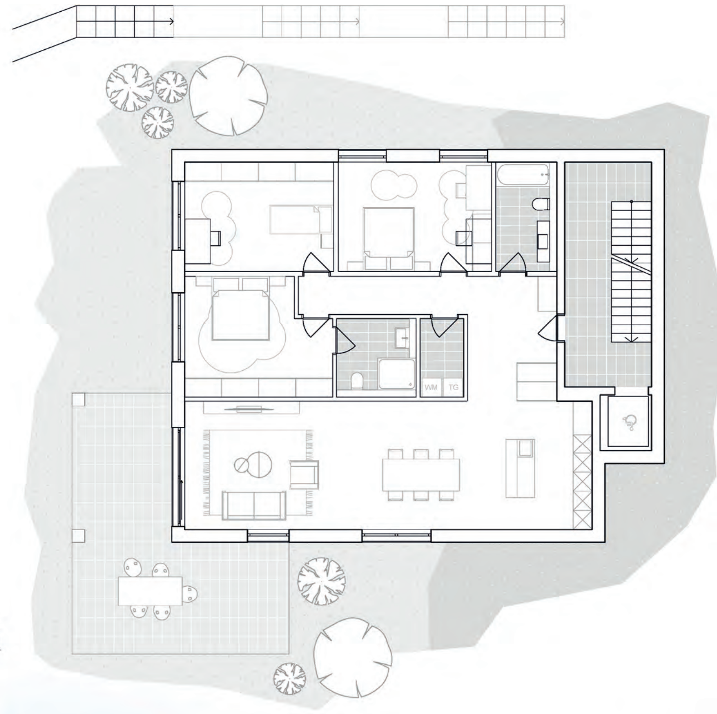
Erdgeschoss
