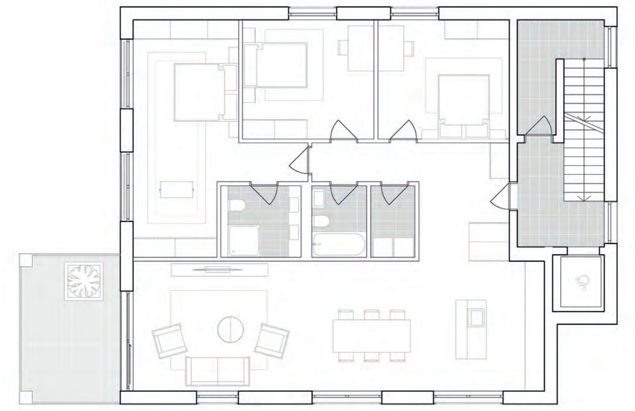
Obergeschoss 2
